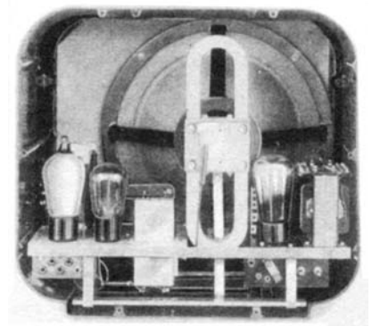
Neufeldt & Kuhnke bleibt beim beliebten Farrand-Inductorlautsprecher und baut ihm ins Gehäuse einen Wechselstromzweier ein.
