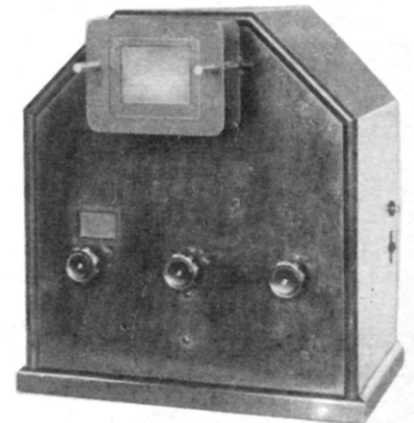
Nipkowscheiben - Projektionsempfänger für 4800 Bildpunkte der Fernseh A. G.
